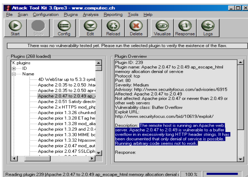
Slika 3.5. Prozor za odabir modula u ATK-u
